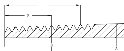
Fig. 3. (Taper)
